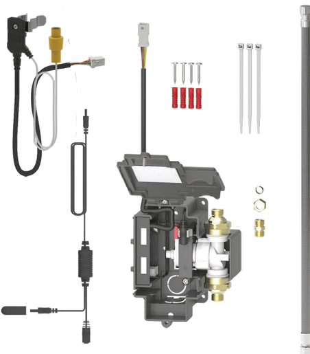
Less Power Sans alimentation Menos potencia
